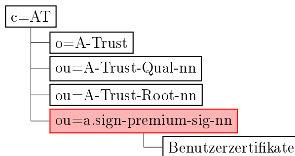
Abbildung 1: A-Trust Verzeichnisbaum
